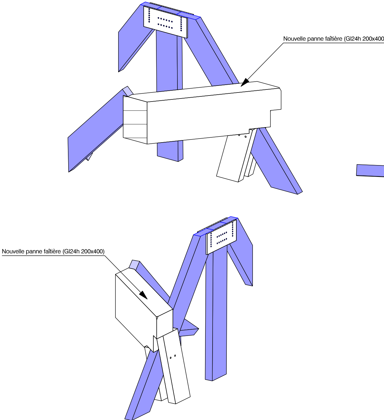
Appuis nouvelle faîtière Ech. : 1:20
