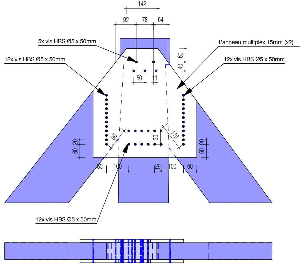
DET.04 Ech. : 1:10
