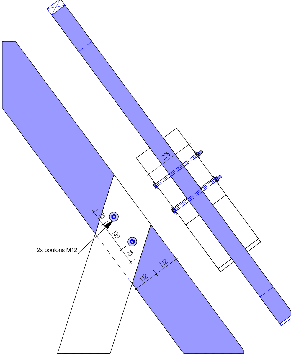
DET.06 Ech. : 1:10
