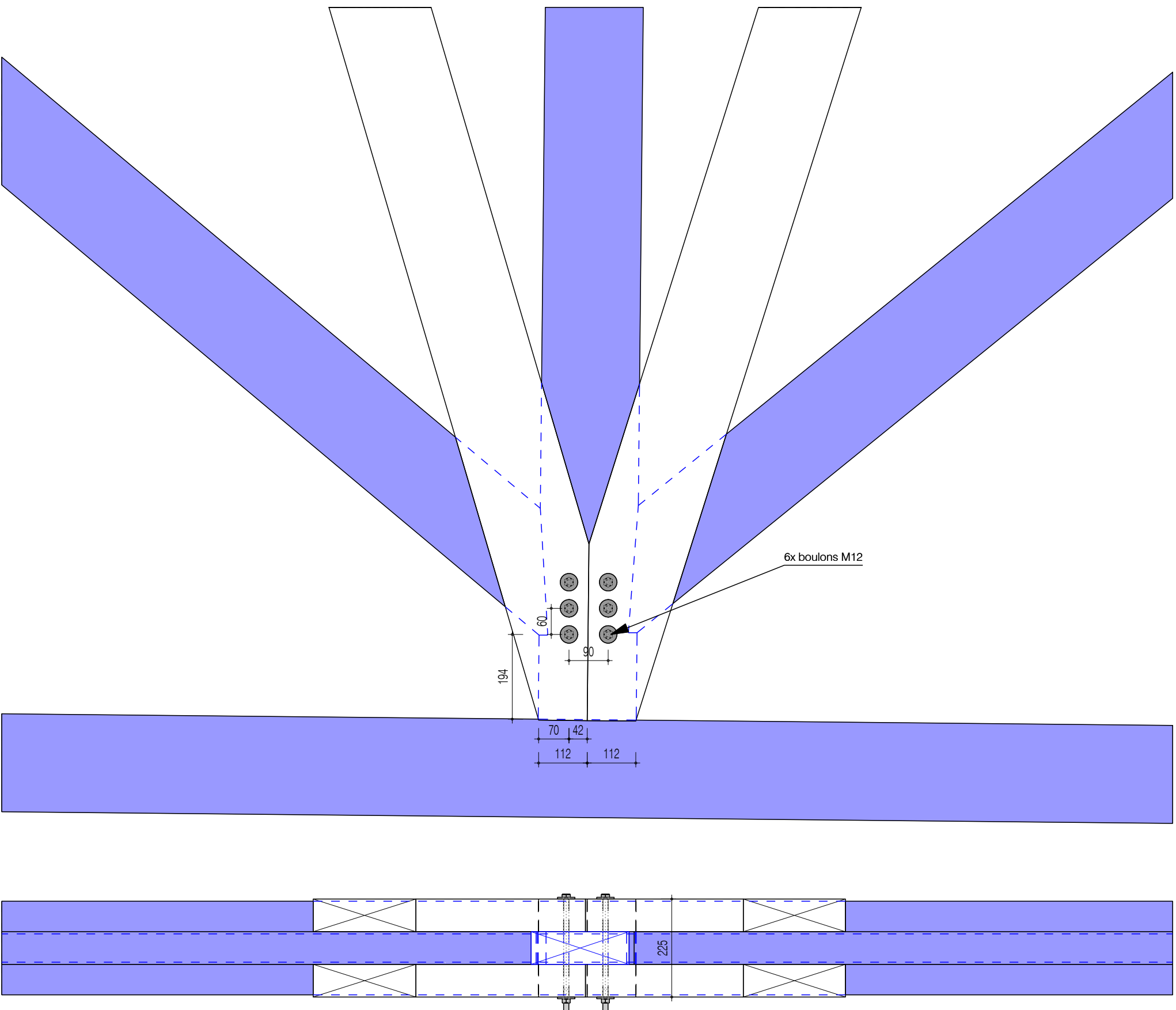
DET.05 Ech. : 1:10
